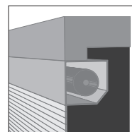
Pose en tunnel intérieure
