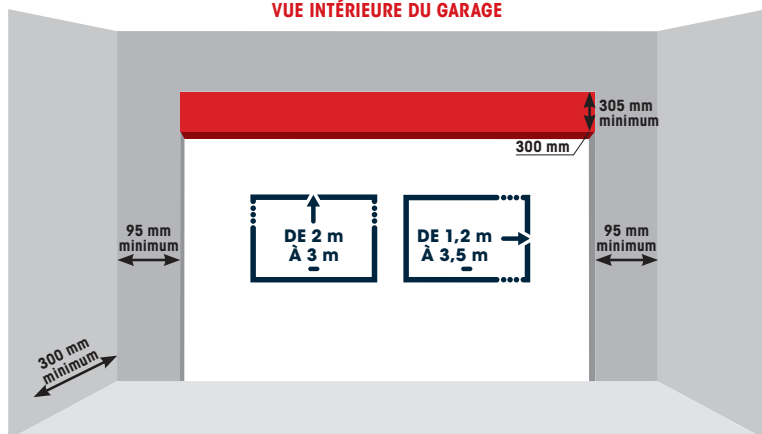
Pose en applique intérieure
